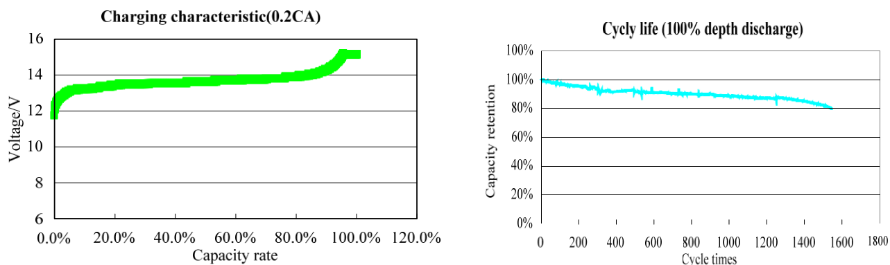
图1 性能曲线图
